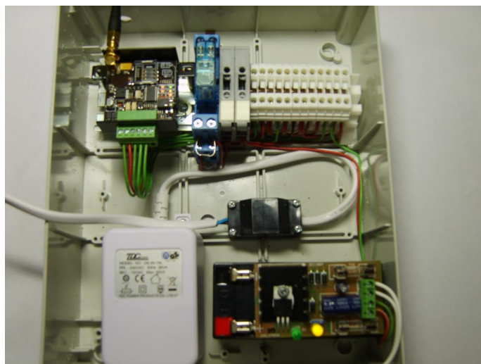
Celé zařízení komunikátoru GSM
